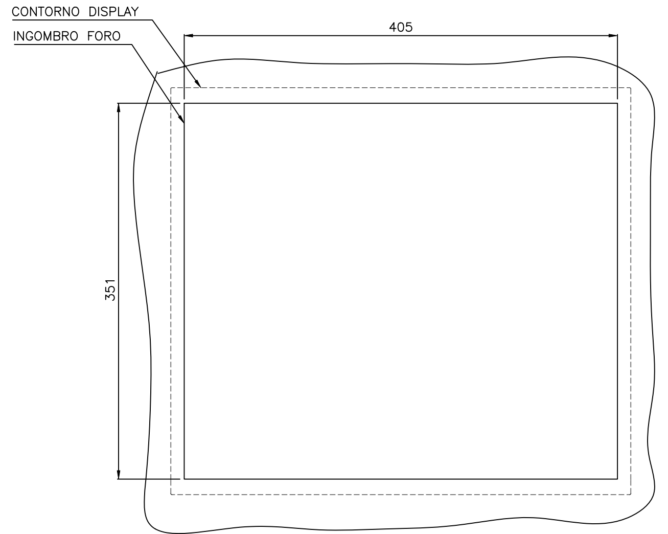
DIMA FORATURA PANNELLO
