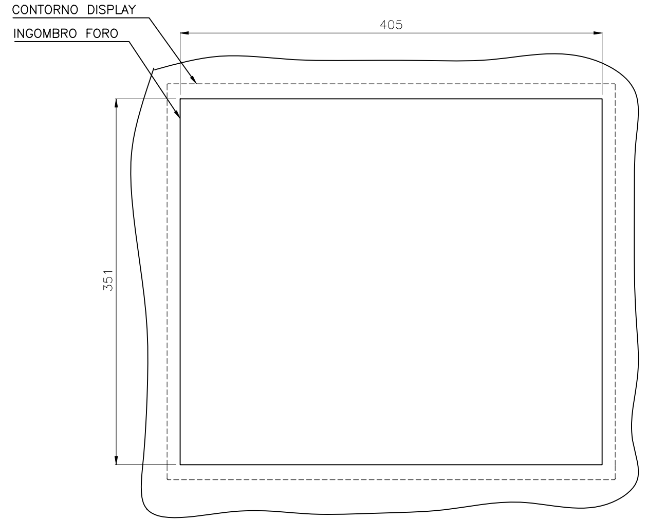
DIMA FORATURA PANNELLO
