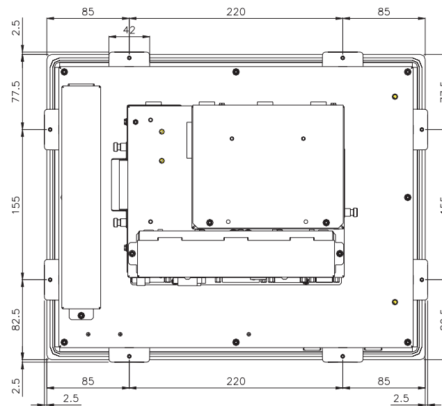
VISTA POSTERIORE Posizione dei ganci di fissaggio
