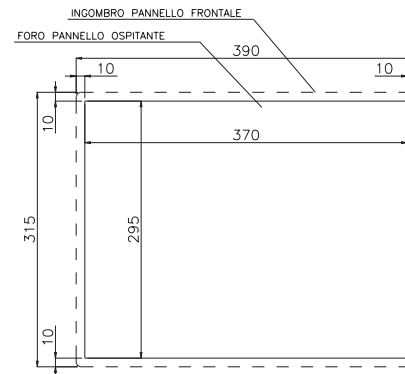
DIMA DI FORATURA PANNELLO
