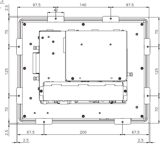
VISTA POSTERIORE Posizione dei ganci di fissaggio
