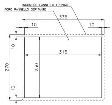
DIMA DI FORATURA PANNELLO
