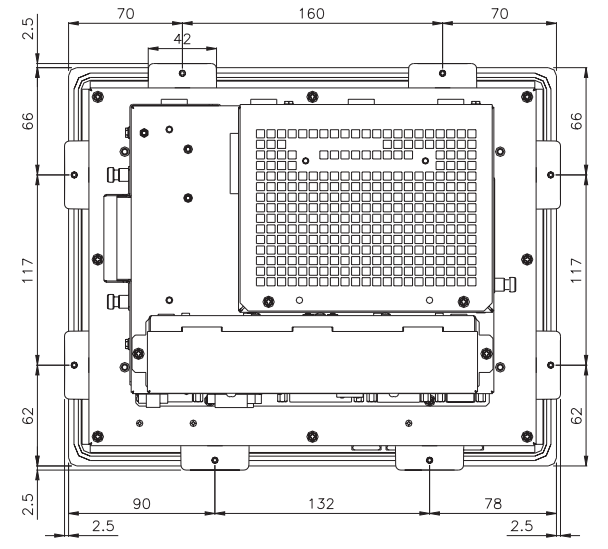
VISTA POSTERIORE Posizione dei ganci di fissaggio
